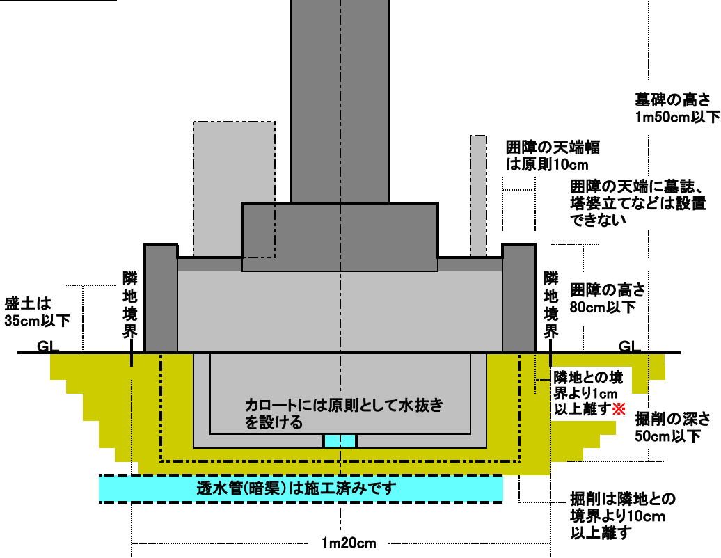
正面図
