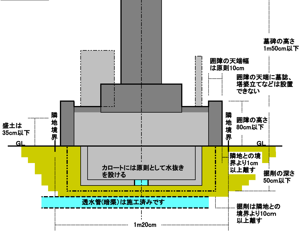
正面図
