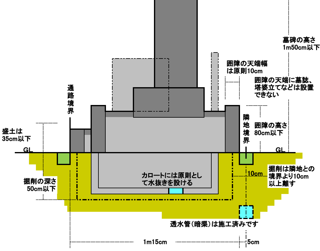
横断面図
